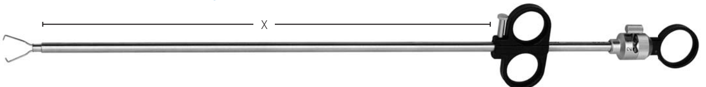
Ringapplikator zur Verwendung durch Trocarhülse Ring applicator for using with trocar sleeve Aplicador de anillo para el uso de operación a través de trocar manga
